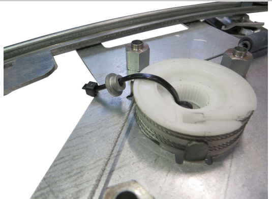
FASCETTA CON ATTACCATA LA GHIERA FORNITA. CLAMP ATTACHED TO THE FASTENER SUPPLIED. COLLIER AVEC LA FRETTE FOURNIE. SCHELLE MIT BEILIEGENDER RINGMUTTER. ABRAZADERA CON EL ANILLO PROPORCIONADO. ABRAÇADEIRA JUNTO COM A COROA FORNECIDA.
