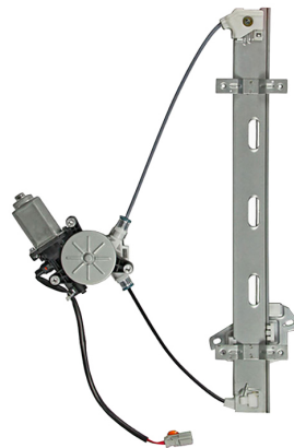
POWER WINDOW RIGHT ALZACRISTALLI ELETTRICO DX
