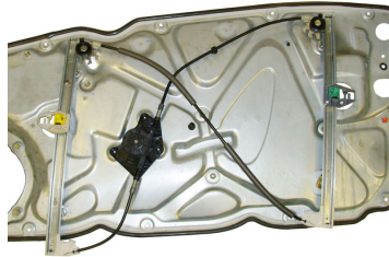
POWER WINDOW LEFT ALZACRISTALLI ELETTRICO SX
