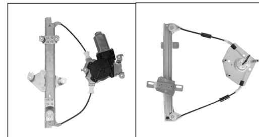
Alzacristallo originale - oem window regulator - lève-vitre original - Fensterheber von oem - elevavinas original - levantador de vidro original - orijinal cam acacagi - Γρύλος γνήσιος
